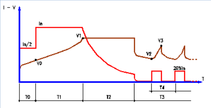
Fig.1: Grafici curve di carica disponibili su macchine PSW e ZHF
